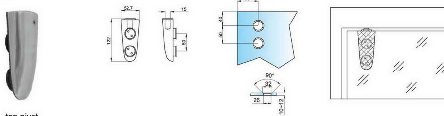
top pivot
