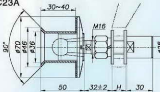
TC23(原代号Original Code:TC21) TC23A
